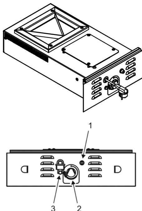
Figura 5 Módulo térmico con elementos de mando
